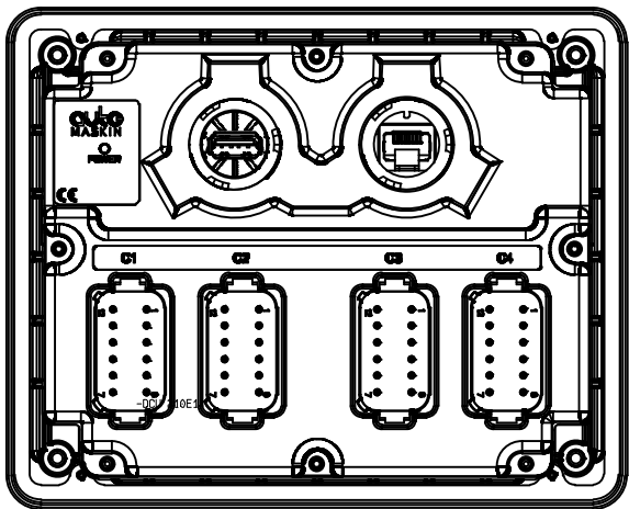
DCU 210E BACK
