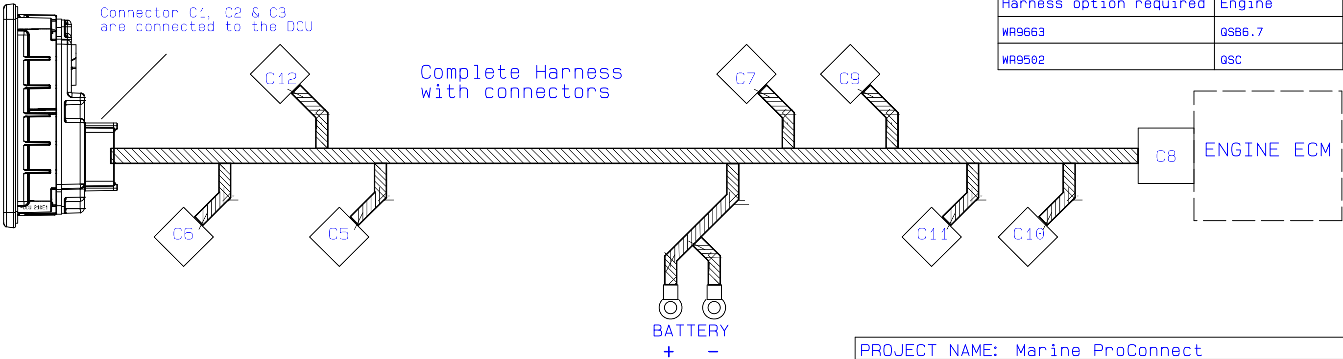
DCU 210E SIDE
